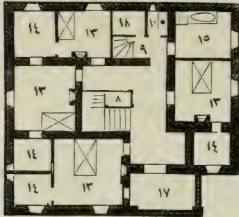
( برنجی قات پلانی )
